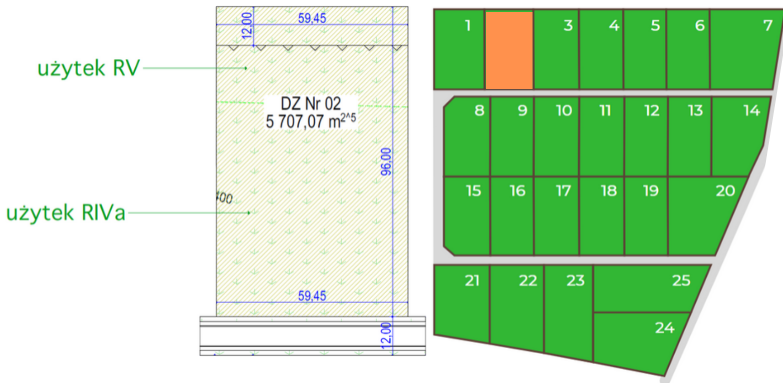
PARAMETRY DZIAŁKI
